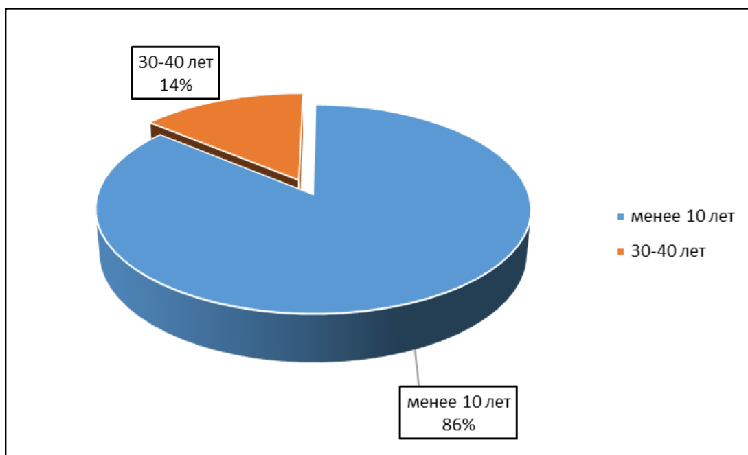
Рис. 2.7. Анализ срока службы силовых трансформаторов АО «Международный аэропорт «Краснодар»
