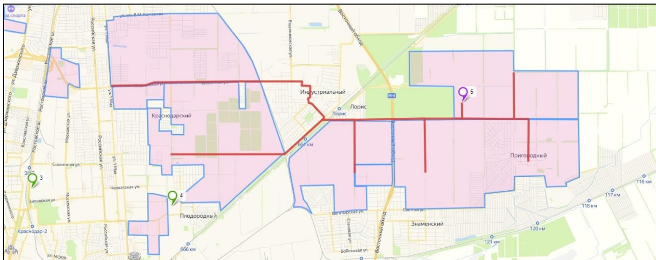
Рис. 3.5. Предварительная схема расположения ТЭЦ и магистральных тепломагистралей в Восточном районе города
